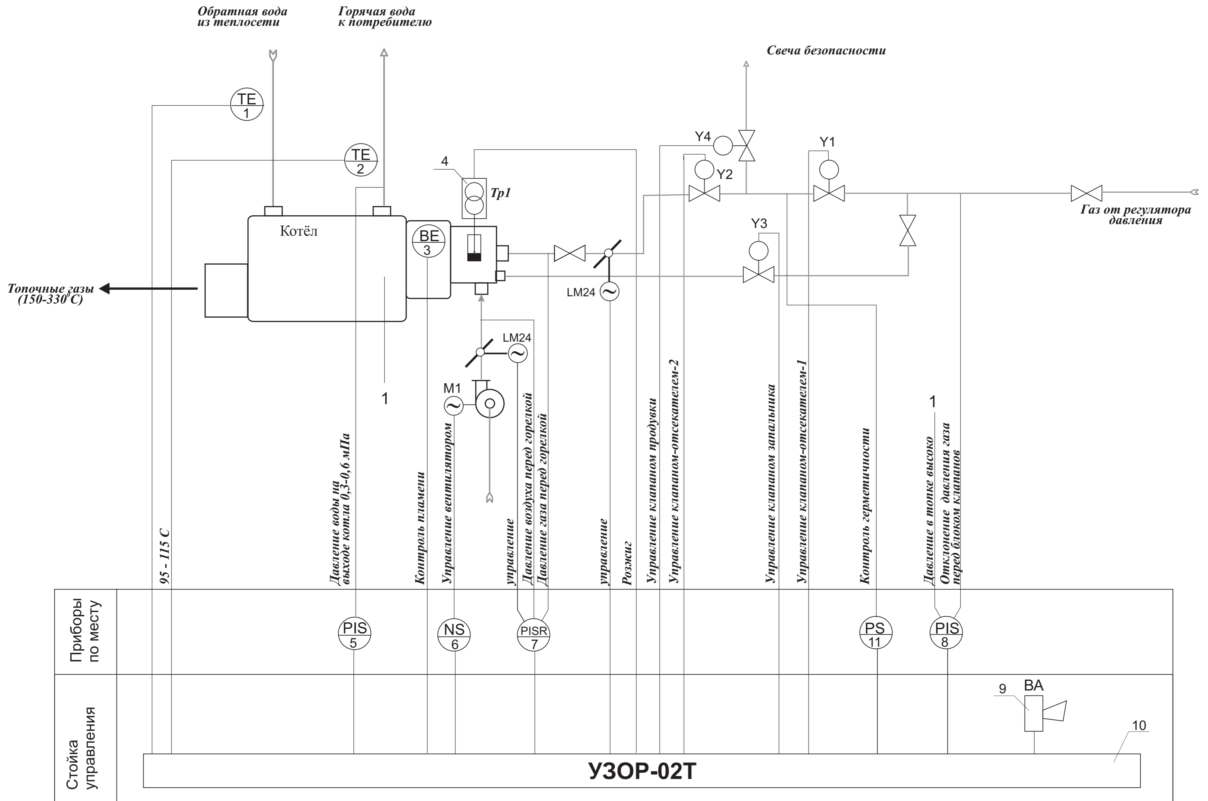
ПРИЛОЖЕНИЕ 1 СХЕМА ФУНКЦИОНАЛЬНАЯ АВТОМАТИЗАЦИИ
