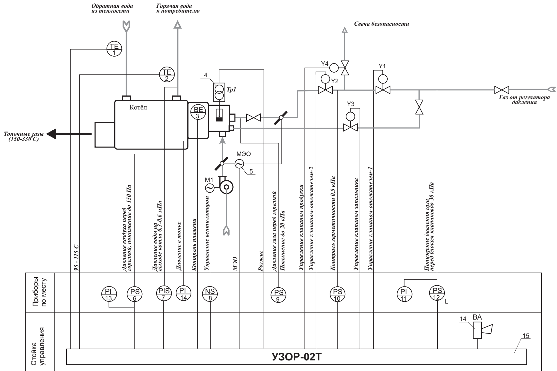
ПРИЛОЖЕНИЕ 1 СХЕМА ФУНКЦИОНАЛЬНАЯ АВТОМАТИЗАЦИИ
